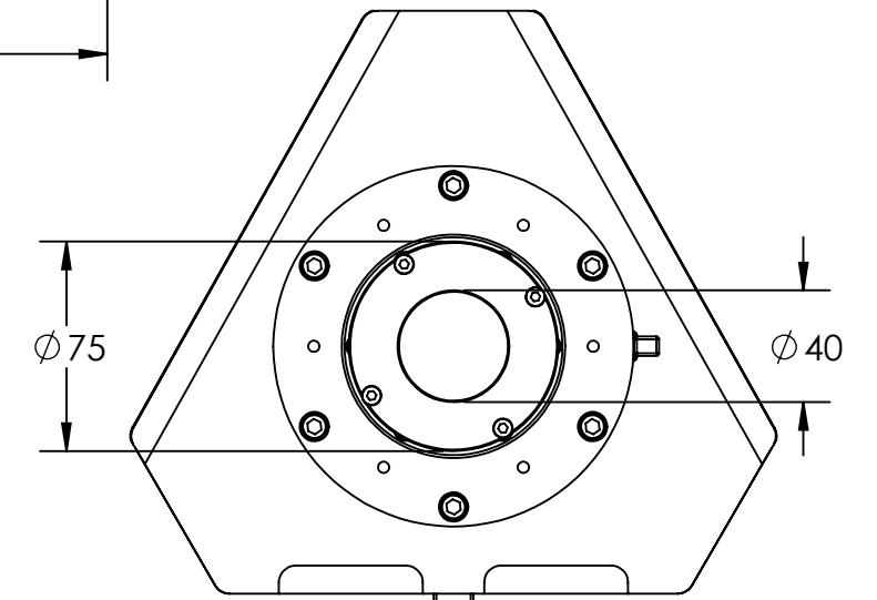
VIEW A-A
